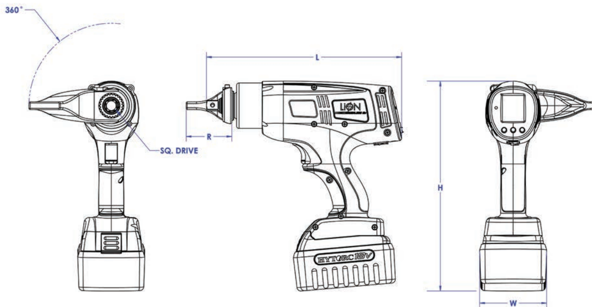
Dimensions du LION Gun
