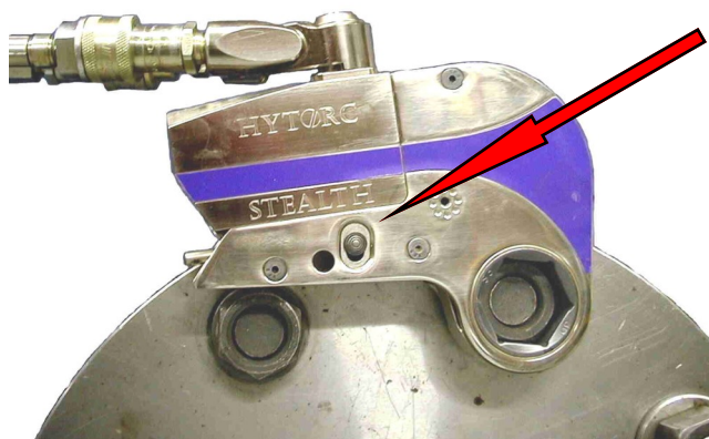
Lever de débrayage
